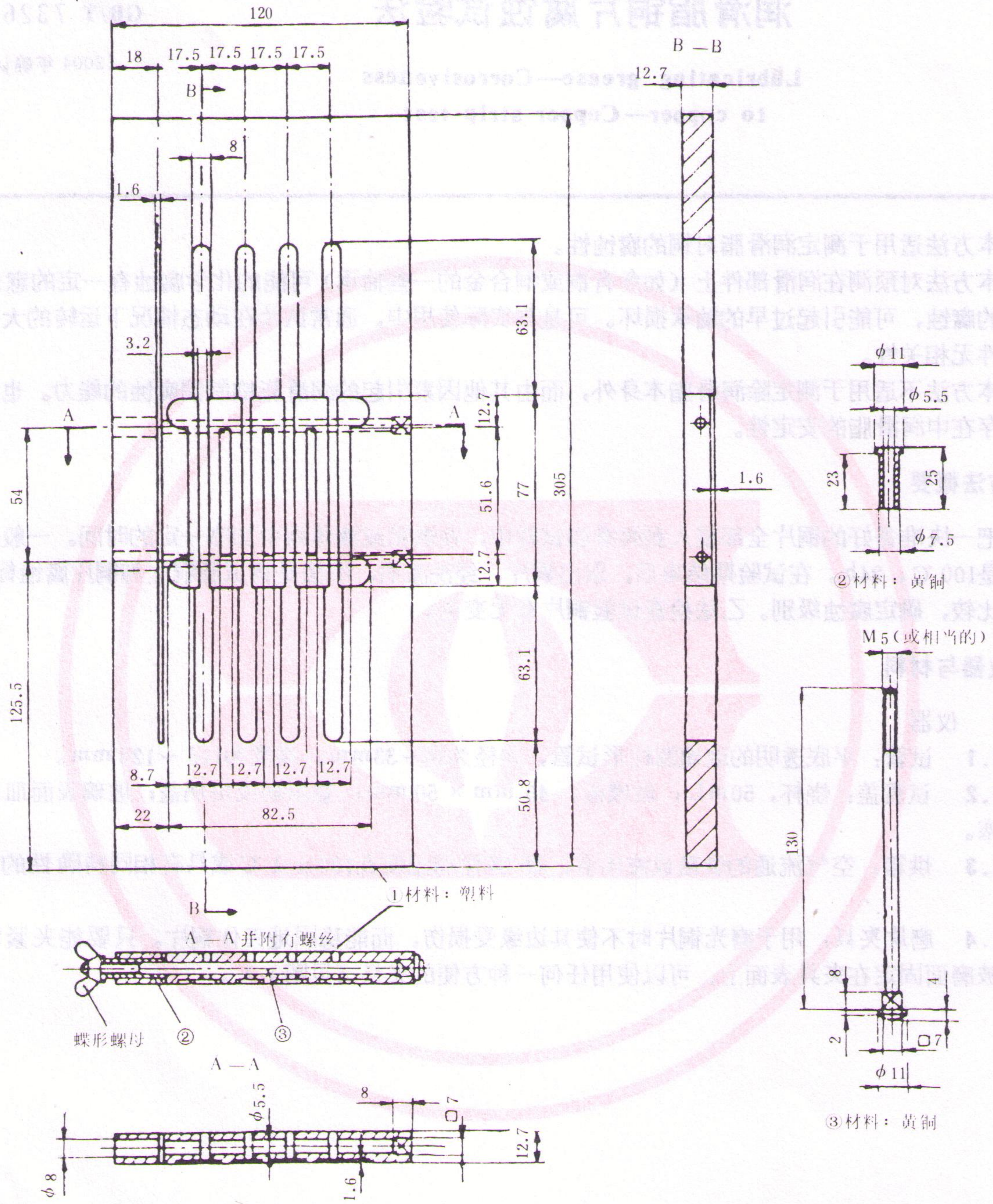
图 1 磨片夹具
