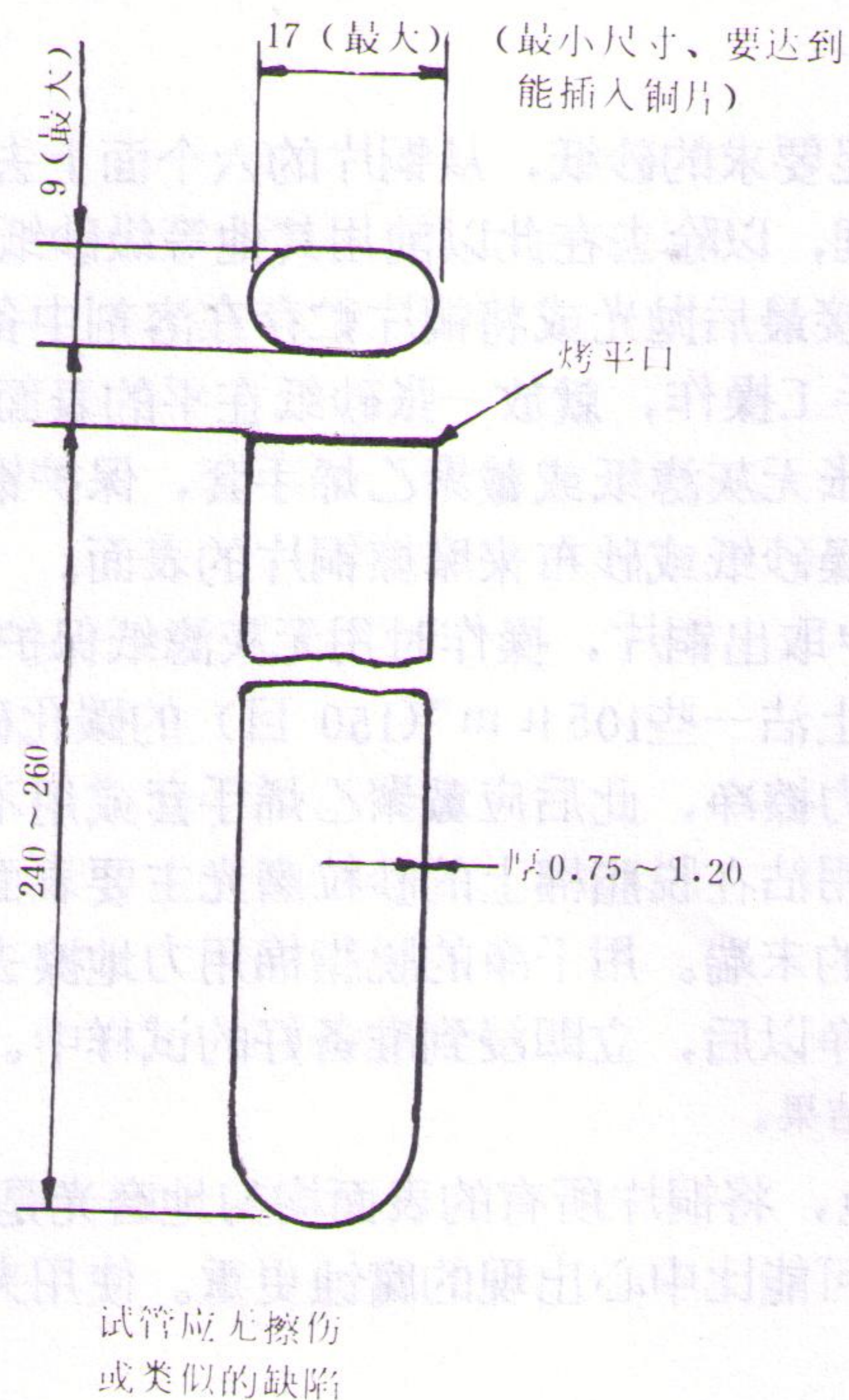
图 2 观察试管
